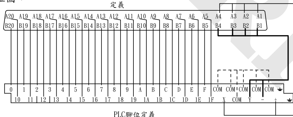
PLC腳位定義
