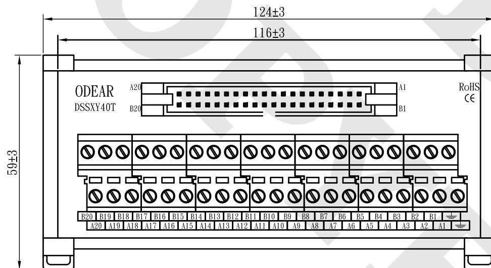
IDC腳位圖：
