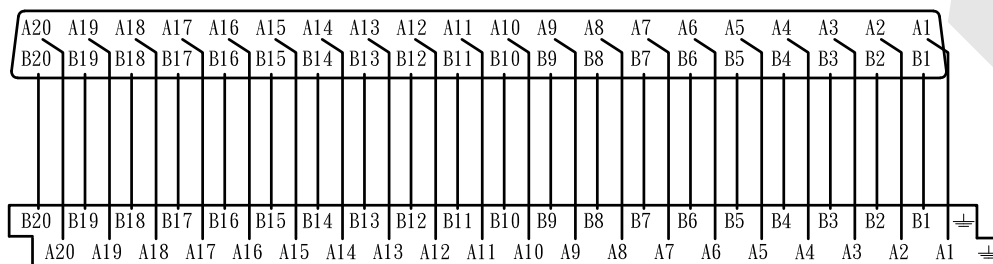
IDC腳位圖：
