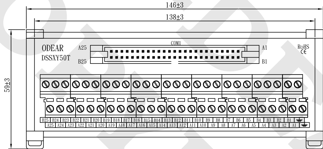
IDC對應腳位圖：
